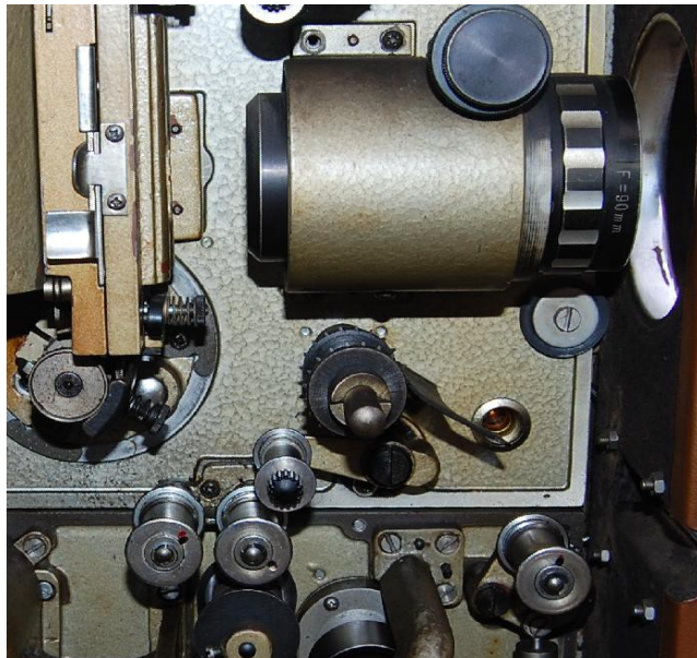
电影放映机
