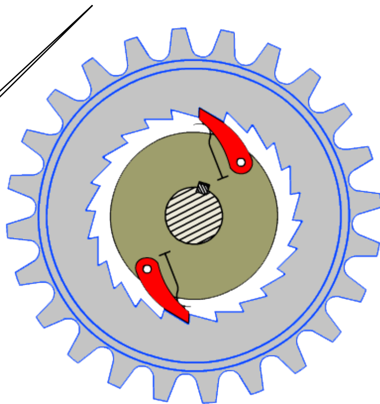
自行车飞轮
