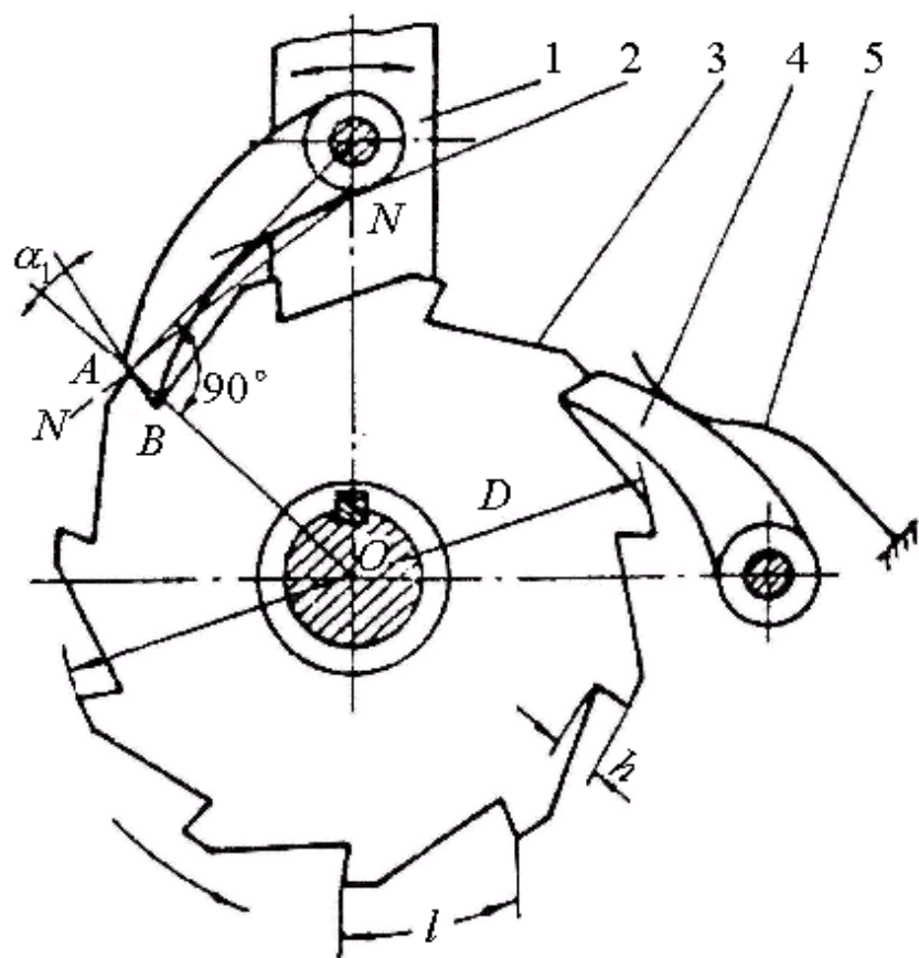
棘轮机构
