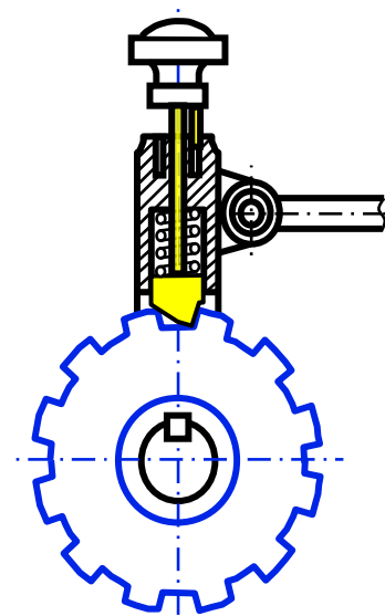
棘轮双向运动2
