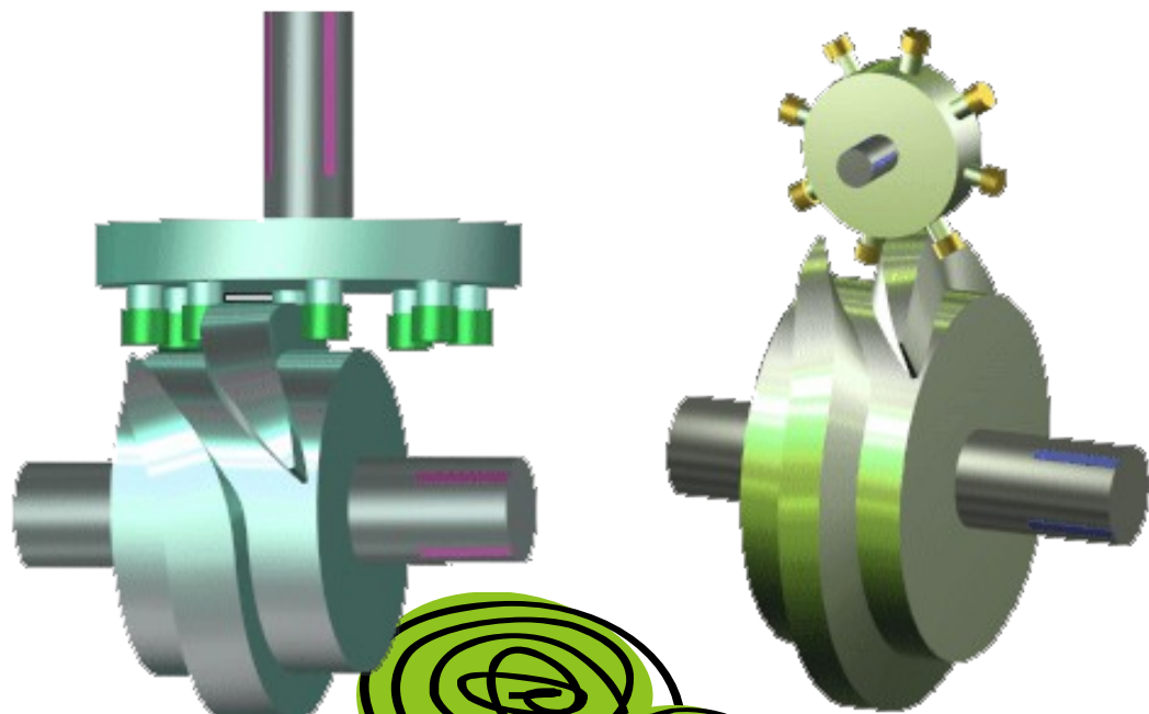
圆柱凸轮间 歇运动机构
