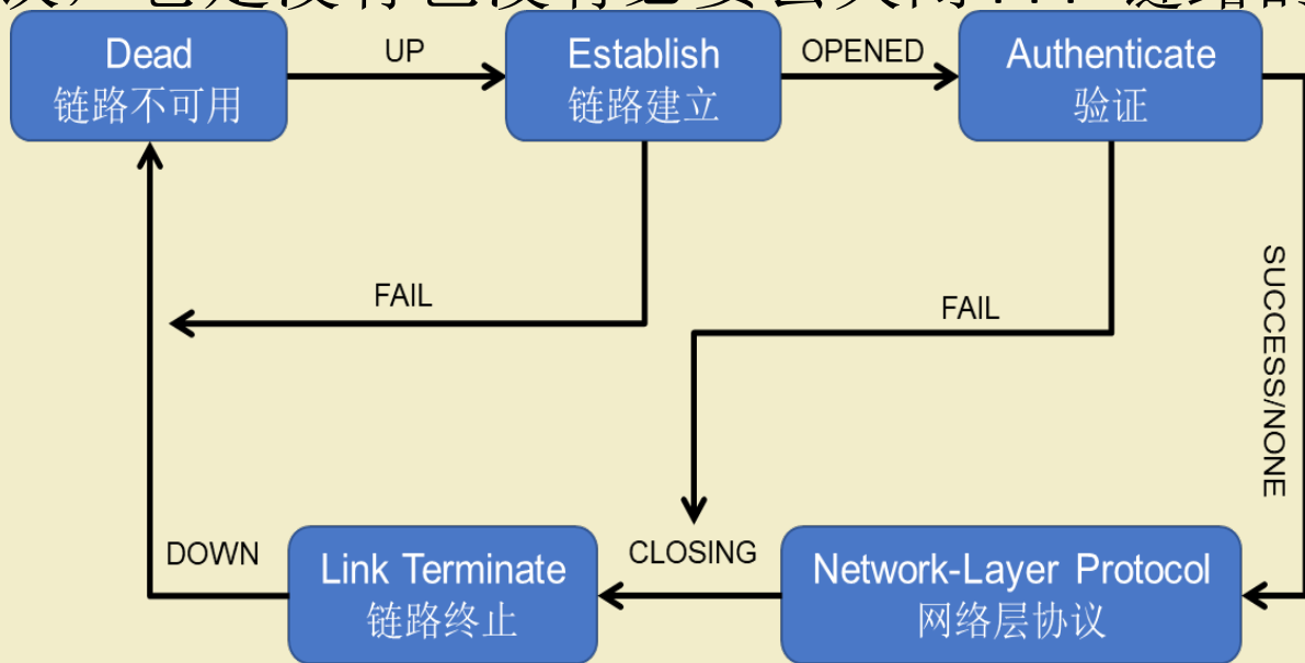
图 9-4PPP 协议过程状态图
