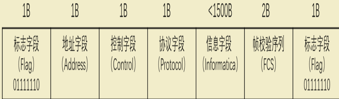
图 9-3PPP 帧的结构
