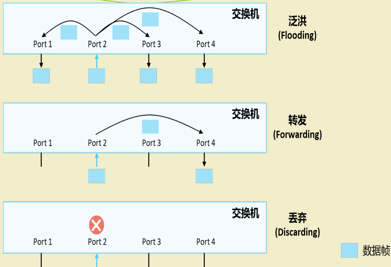
图 2-17 交换机对数据帧的处理行为
