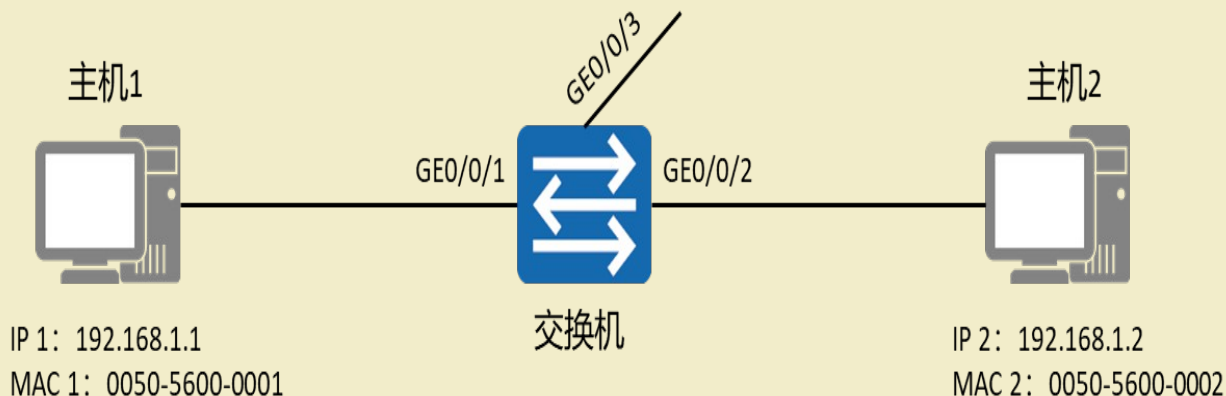
交换机的MAC地址表
