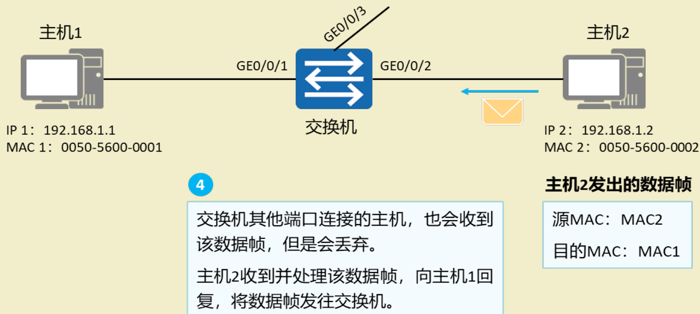
图 2-24 交换机 MAC 地址表的形成过程 4
