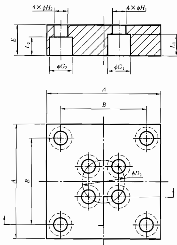
图 2 A2 型固定座板
