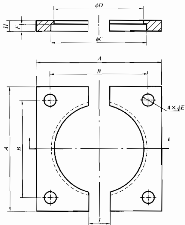
图3 B型两半式固定夹板
