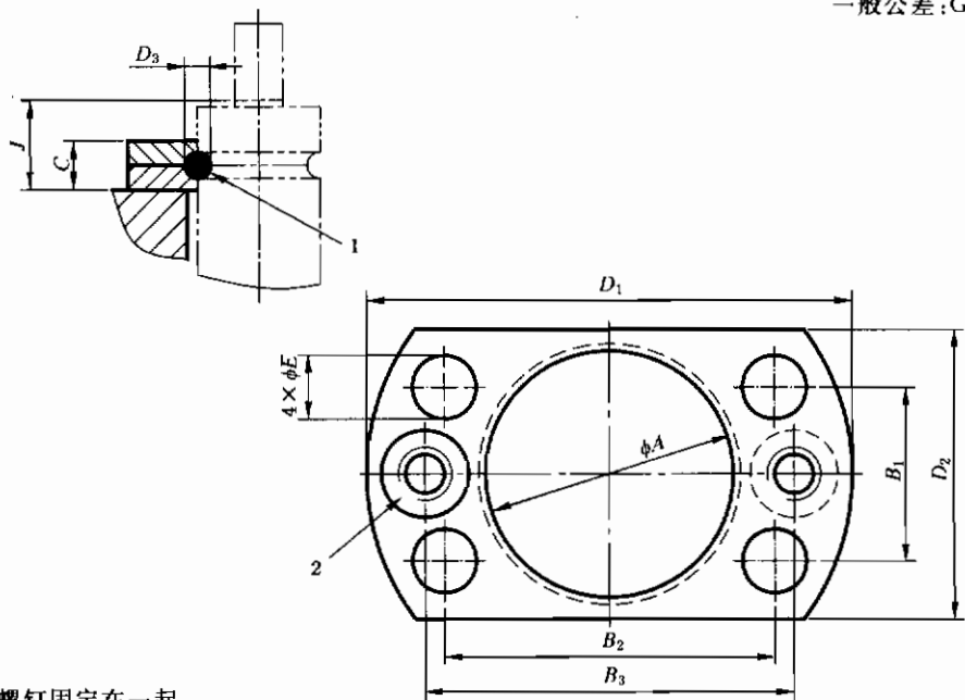
两法兰应用螺钉固定在一起。 1——平卡箍； 2——装配螺钉孔。
