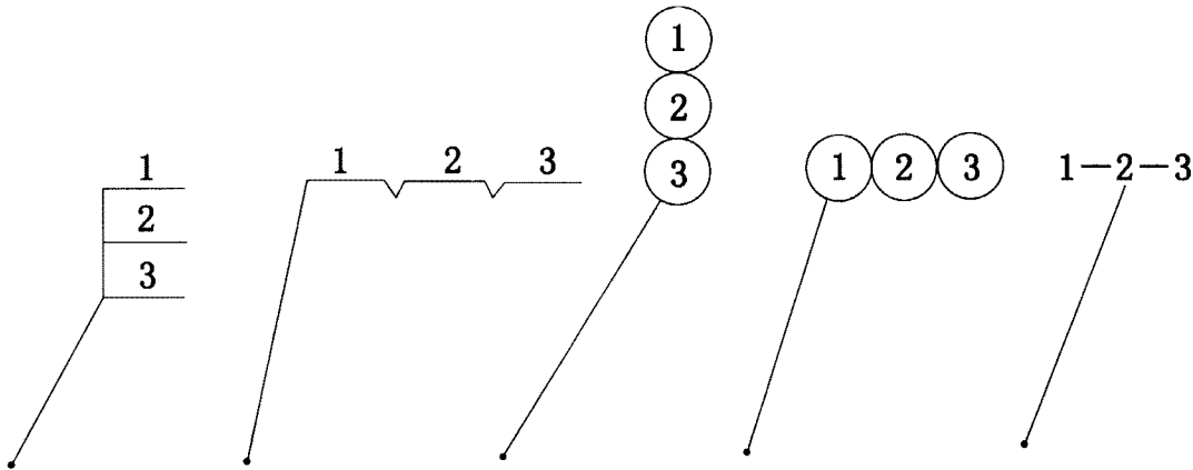
图 3 公共指引线的编注形式
