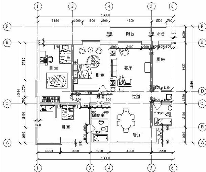
商品房单元平面图 1:100
