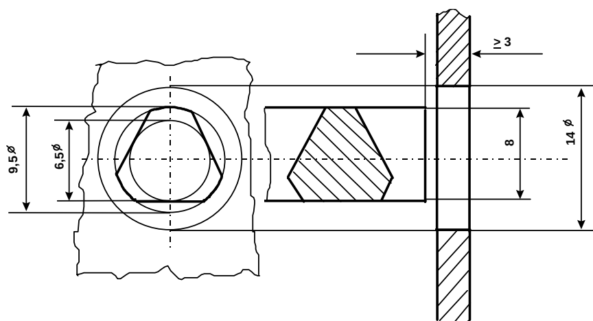
图B1 开锁三角形钥匙
