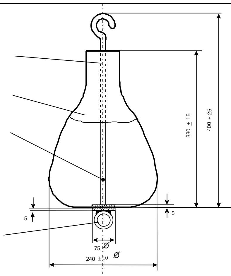
①—螺杆；②—在最大直径的平面内测量跌落高度的参考点；③—皮袋；④—钢制圆盘；⑤—触发装置附件 图 J2 软摆锤冲击装置
