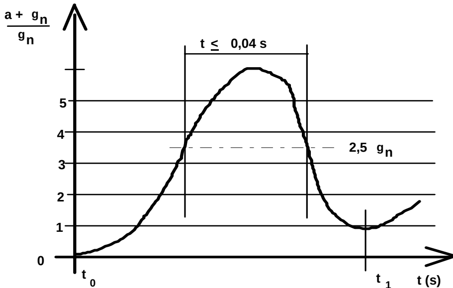
图F1 减速图
