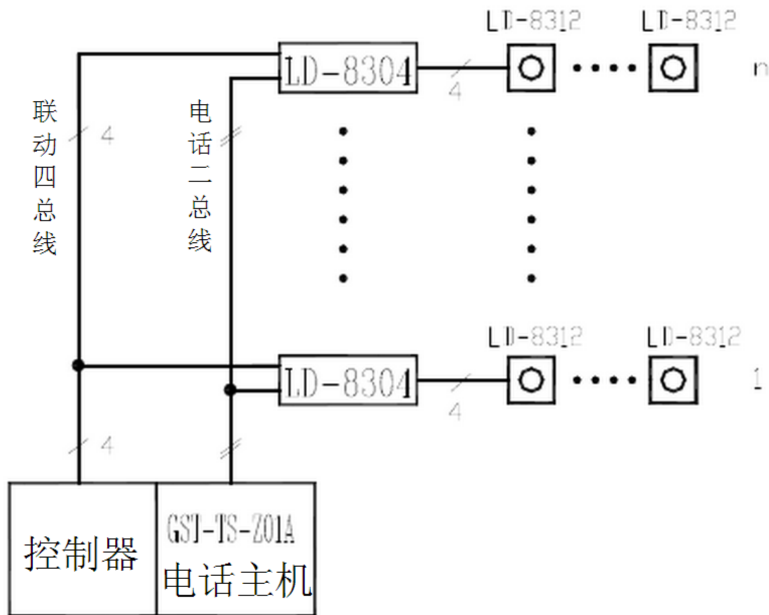
图 3 电话插孔分区编码的系统连接示意图
