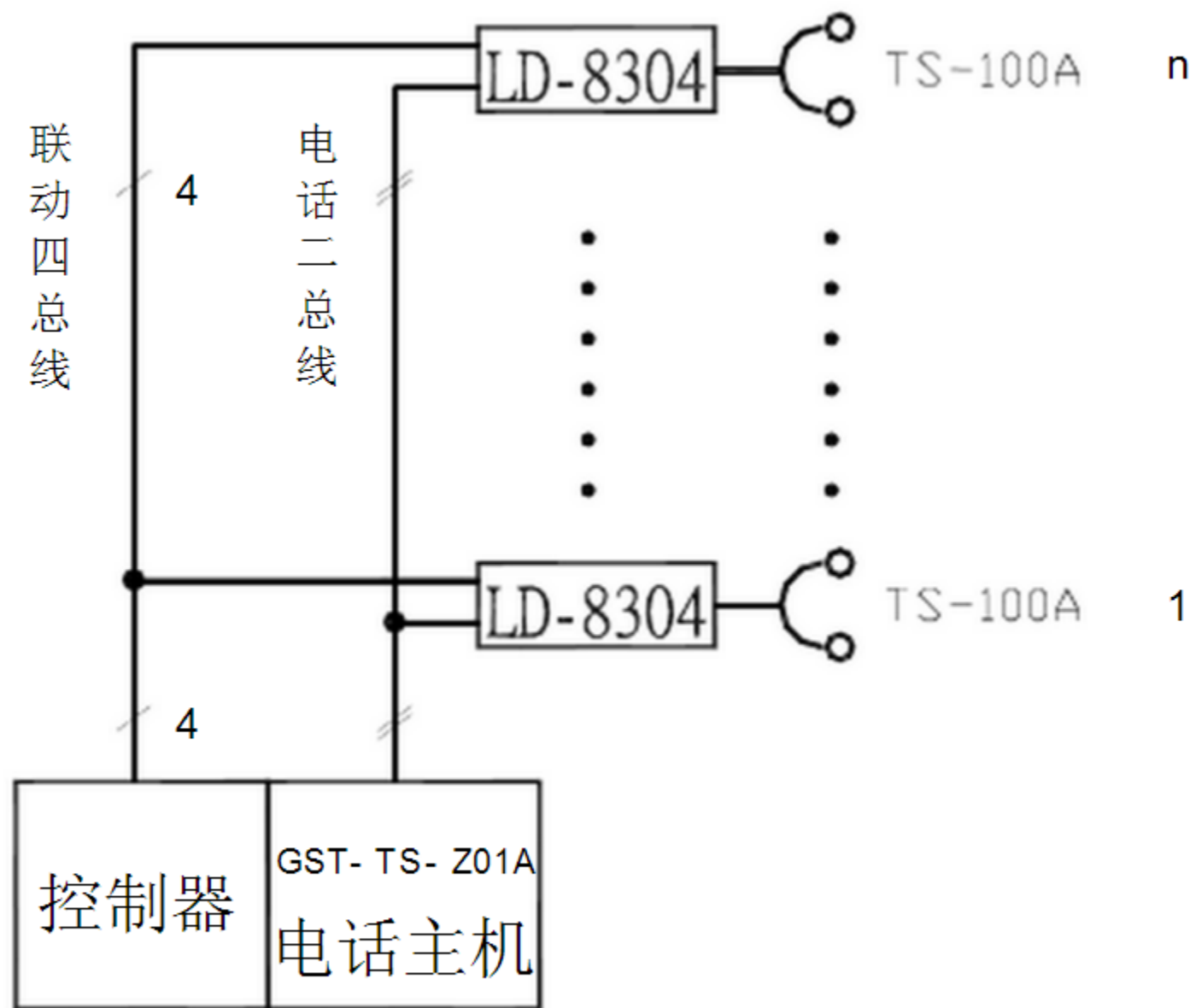
图 2 现场全部为固定式分机的系统连接示意图
